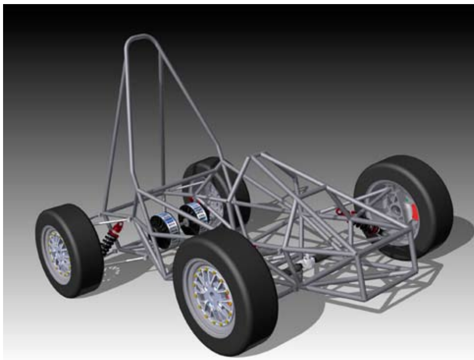
Tölvuteikning af grindinni með fjöðrunarkerfi, mótorum og stýrisbúnaði.
