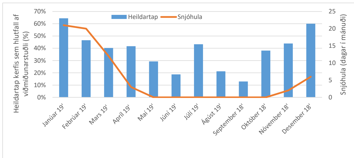
Mynd 7: Heildartap kerfis sem hlutfall af viðmiðunarstuðli. Dagur snjóhulu úr gögnum frá Væðurstofunni (2019).
