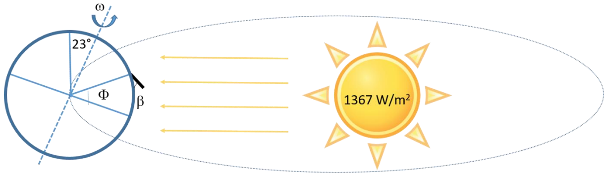
Mynd 2: Inngeislun sólar á hallandi flöt ræðst af breiddargráðu ( \Phi ), hvernig jörðin snýr gagnvart sólu (ræðst af tíma dags og árstíð) og halla flatar ( \beta ) frá láréttnu.
