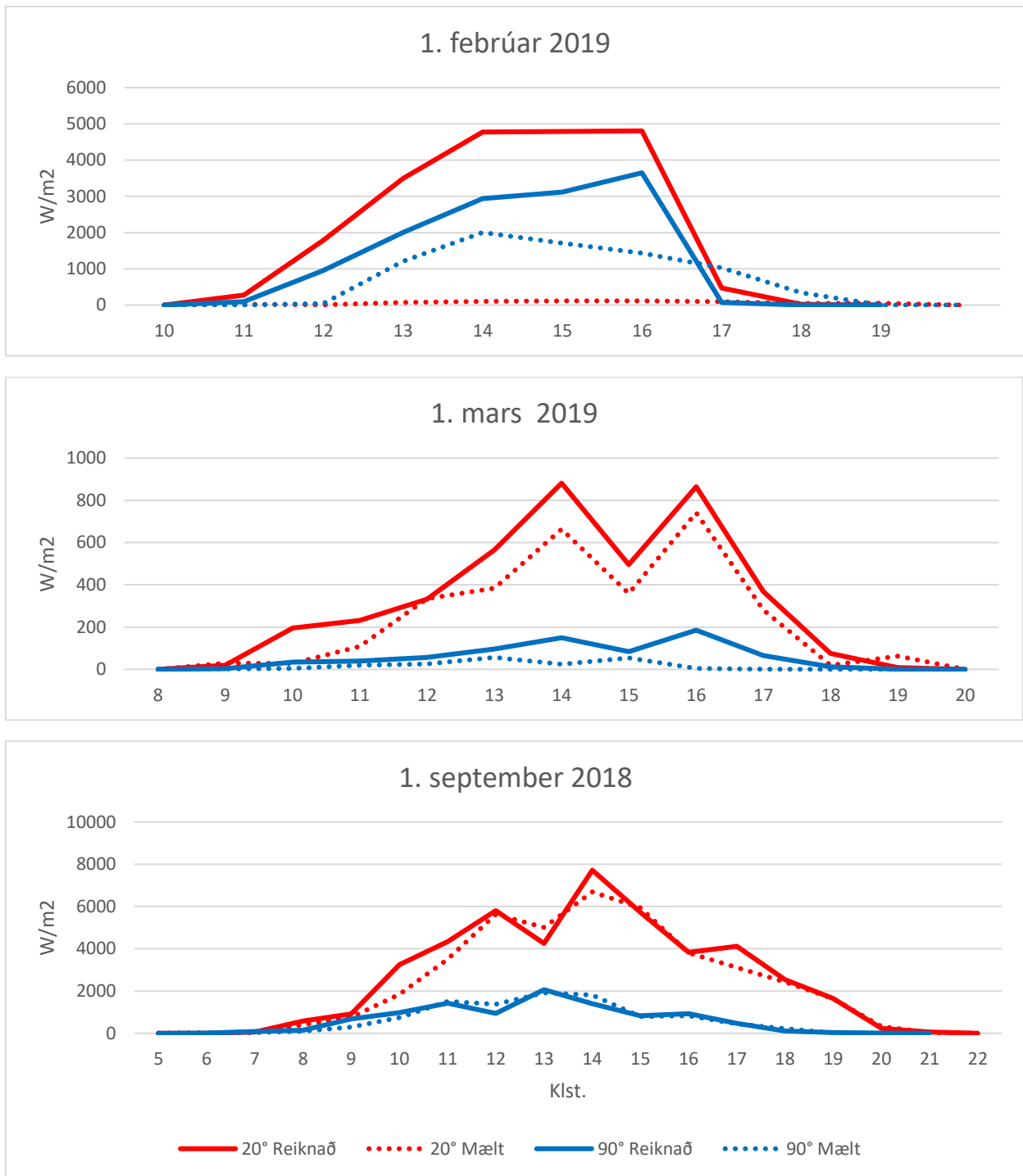
Mynd 3: Samanburður á mældri (heil lína) og reiknaðri (brotalína) sólarinngeslun á þremur dögum.
